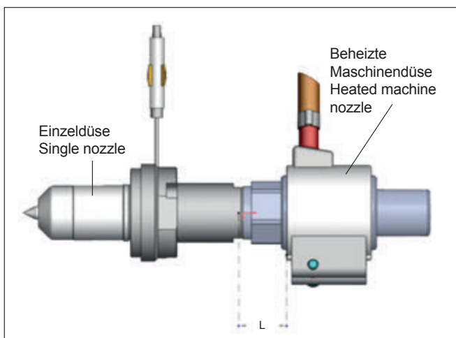
Abb. 1: Einzeldüse mit beheizter Maschinendüse. Das Heizband sollte so dicht wie möglich in Richtung Einzeldüse platziert werden. Fig. 1: Single nozzle with heated machine nozzle. The heating tape should be placed as closely as possible in the direction of the single nozzle.
