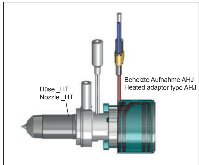
Abb. 3: Düse HT mit beheizter Aufnahme Fig. 3: Nozzle HT with heated adaptor
